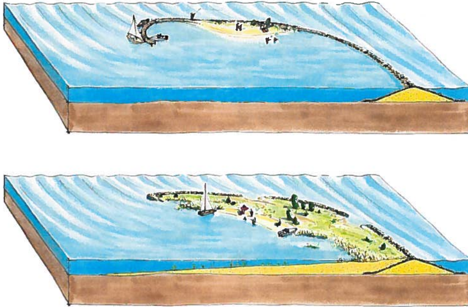
Figuur 4 Visualisatie dwarsdoorsnede voorgesteld voorkeursalternatief (stap 1) en stap 2 (onder) [Stroming]
